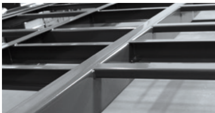
Ganz-Alu-Unterbaukonstruktion
